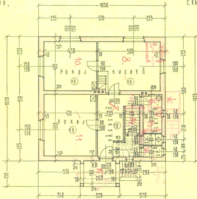
PŘÍZEMÍ 1:100,
