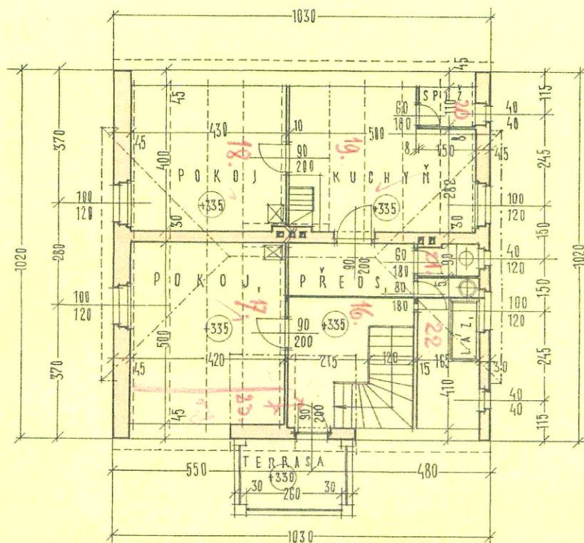
P O D K R O V Í 1:100,
