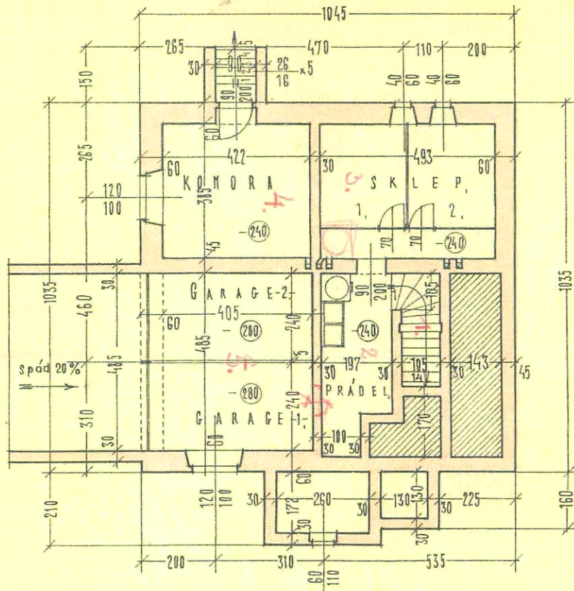
SUTERÉN 1:100,
