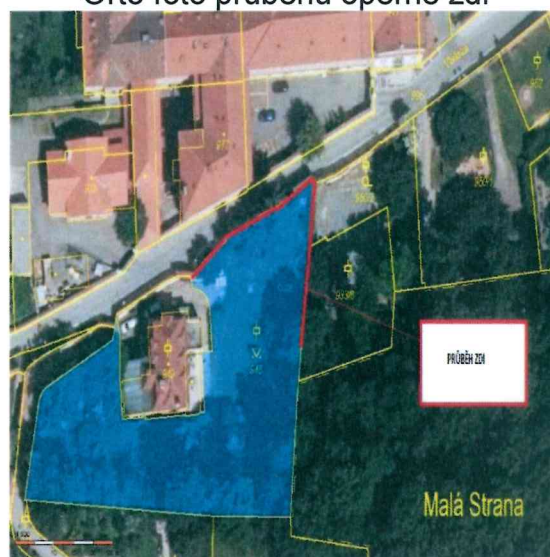
Orto foto průběhu opěrné zdi
